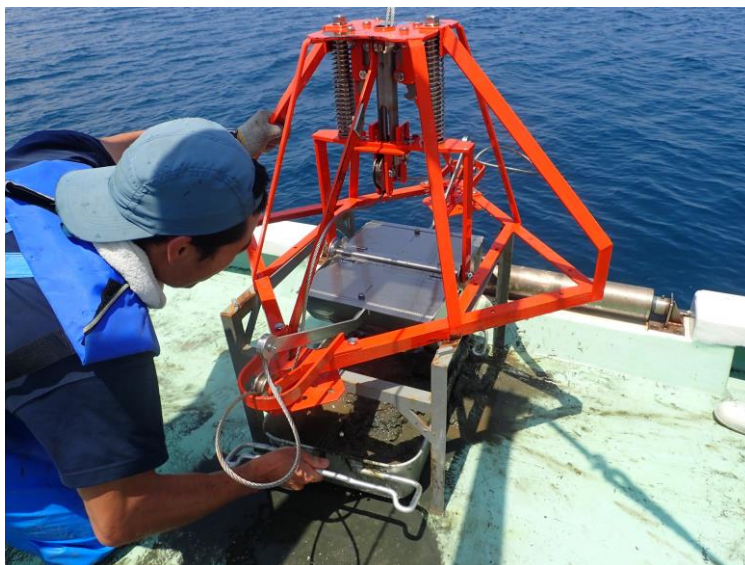
スミス・マッキンタイヤ型採泥器
